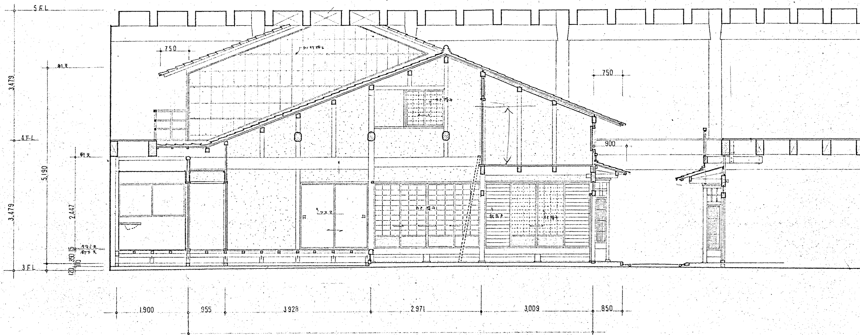
A-A SECTION
